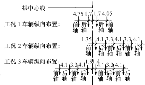
(a) 各工况车辆纵向布置图
