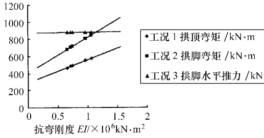
图5 各工况模型桥截面内力随抗弯刚度变化趋势图
