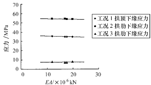
图 4 各工况拱肋下缘应力随抗压刚度变化趋势图
