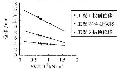
图9 各工况拱肋截面位移随抗弯刚度变化趋势图
