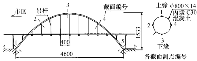
图1 群益大桥总体布置及测点布置图/mm
