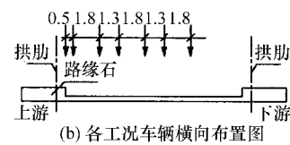
图2 各工况车辆布置图/m
